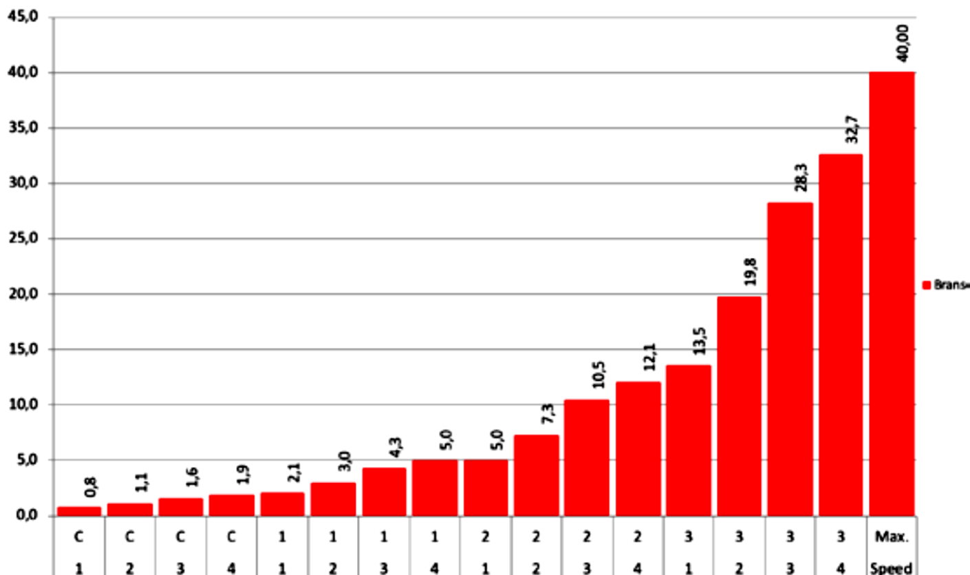
Branson K78 snelheidsgrafiek
