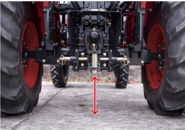
De Branson 00-serie heeft een uitstekende bodemvrijheid.
