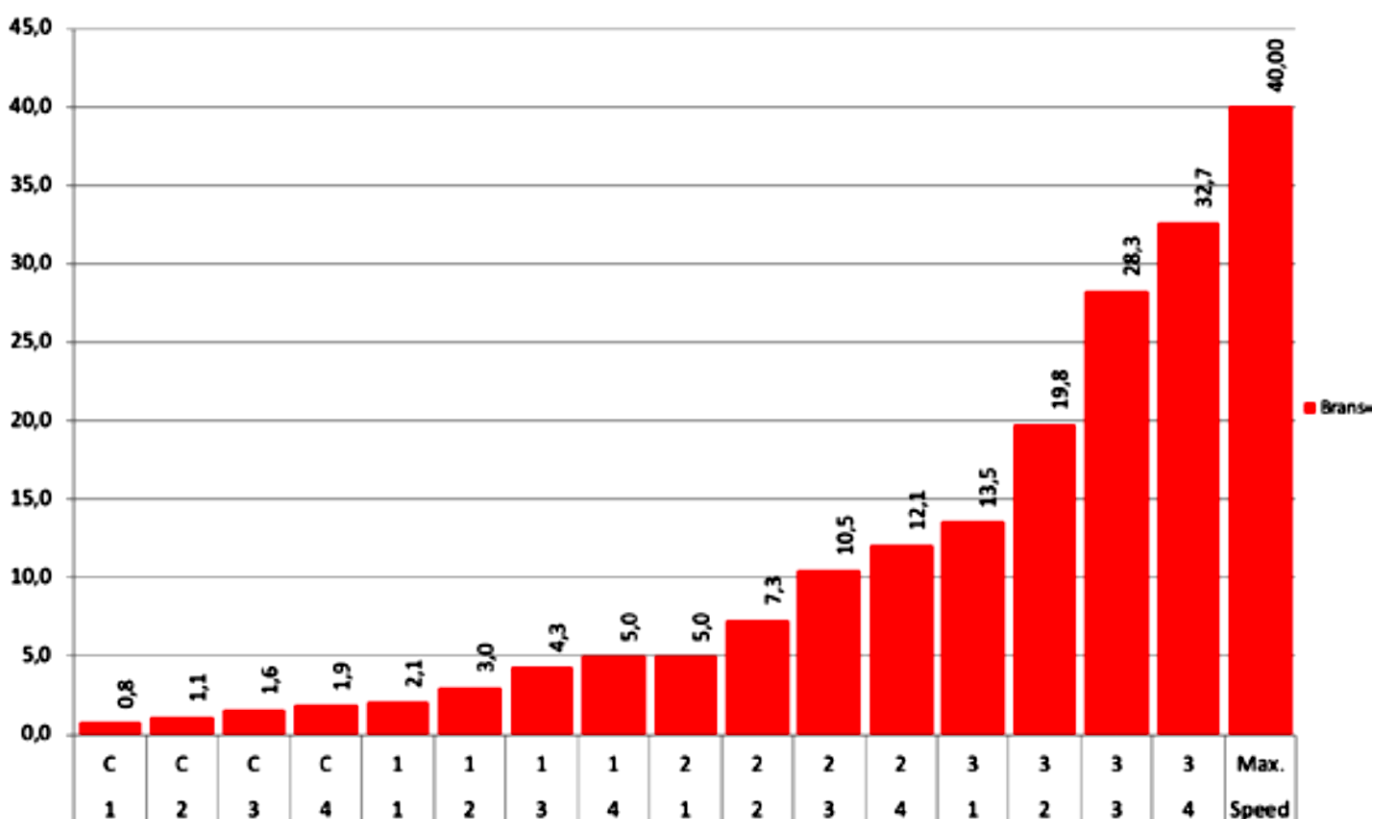
Branson K78 snelheidsgrafiek
