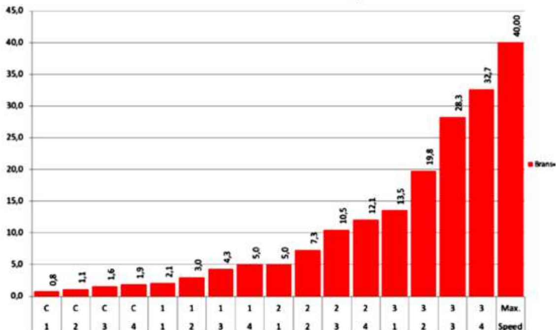
Branson K78 snelheidsgrafiek
