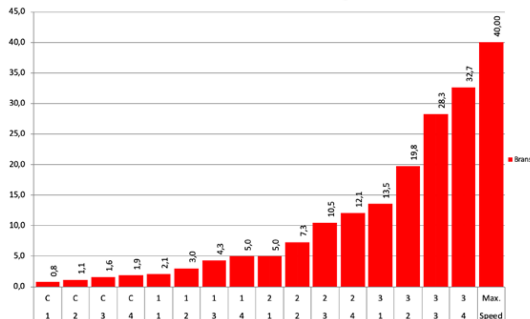
Branson K78 snelheidsgrafiek
